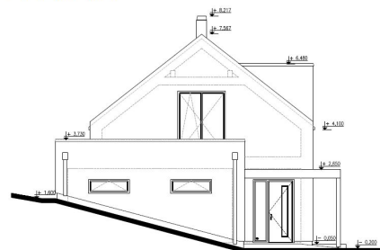
ZÁPADNÍ POHLED
